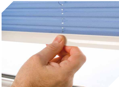
Feszített raffroló – a zsinórok feszítettek, a redőny csak a helyére húzható/tolható
